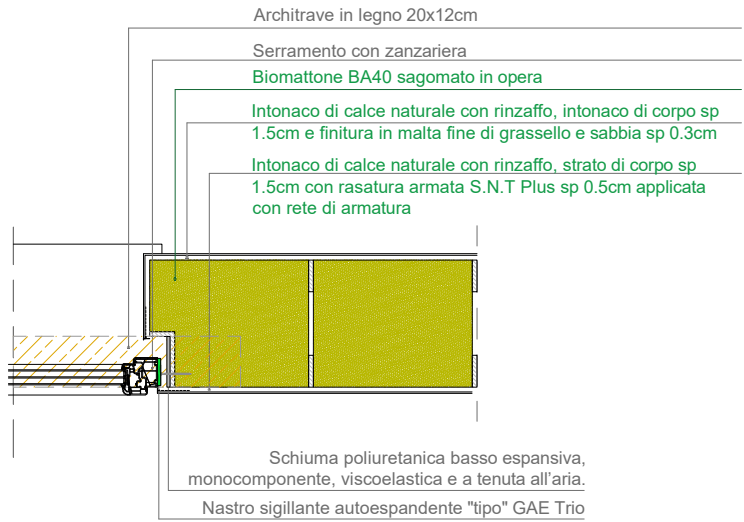
Sezione all'altezza del serramento
