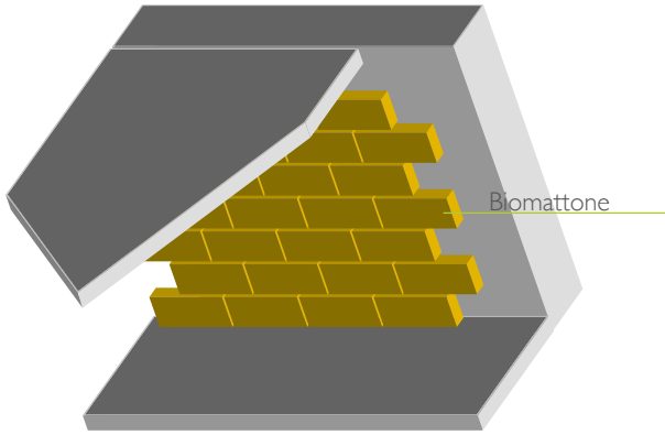
Abb. 3 - Vorgesetzte Dämmschale
