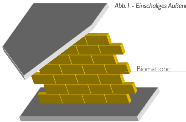
Abb. 1 - Einschaliges Außenmauerwerk
