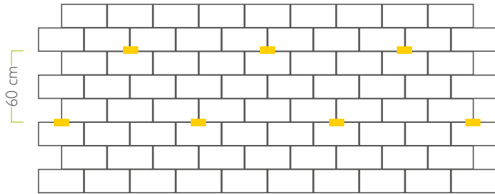
150 cm Verankerungsbild
