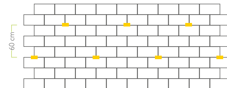
150 cm Verankerungsbild Verankerungsdetail Biomattone® auf bestehender Wand
