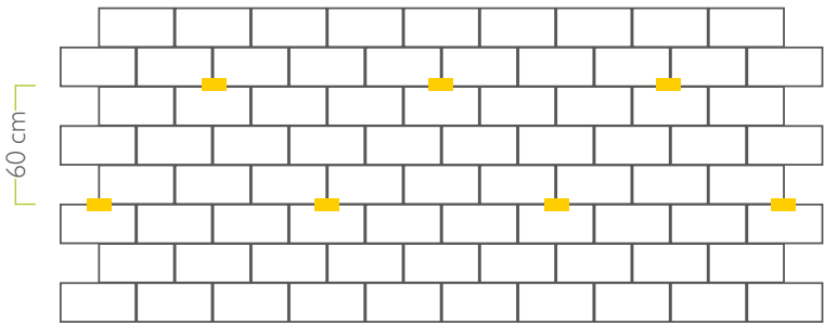
150 cm Prospecto Final Detalle anclajes Blocco Ambiente® falsas paredes existentes
