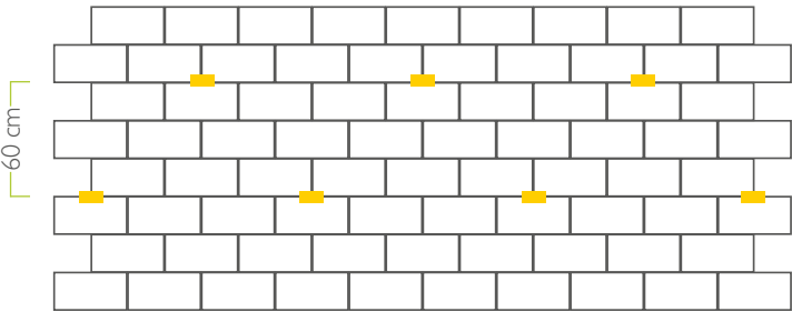
Fig.4 Detalle anclajes Ladrillos ecológicos falsas paredes
