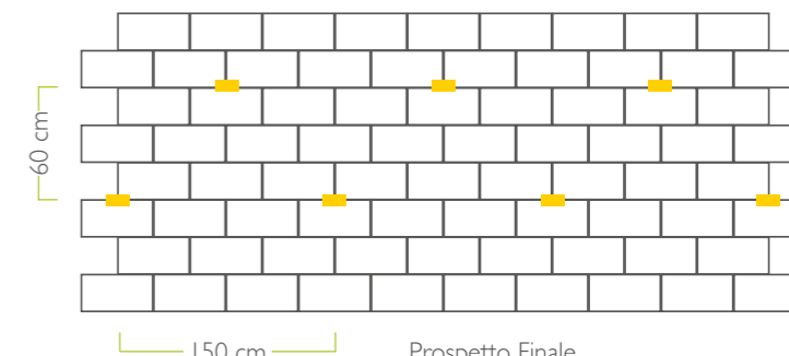
Fig.4 Dettaglio ancoraggi Biomattone contro muri esistenti
