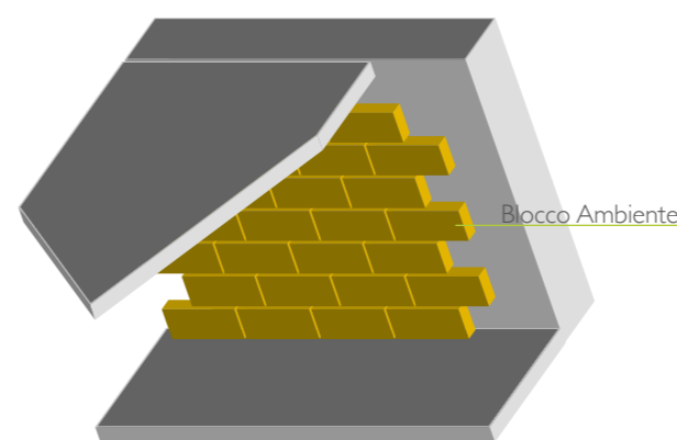
Fig.3 Controparete isolante
